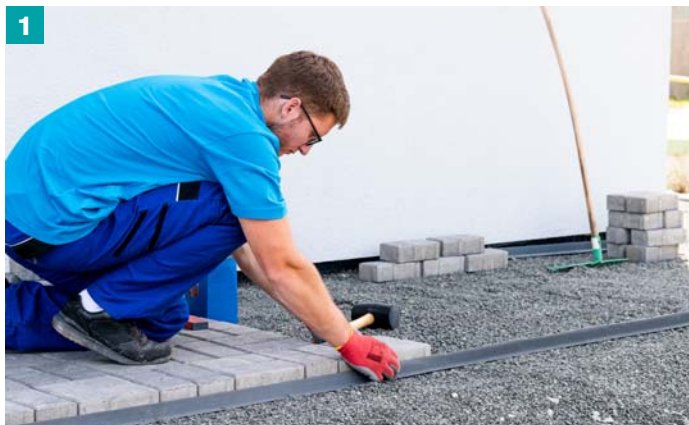
1 Ukončovací profil RET-FIX osadíme na místo určené pro instalaci dlažby.
