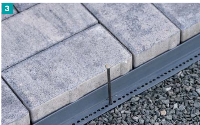
3 Ukotvíme jej ocelovými hřebíky, množství kotvení je asi 5 hřebů na jeden metr.
